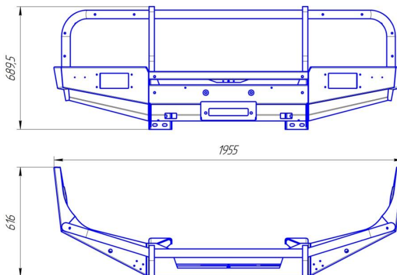
Рис. 3 Габаритный чертёж
